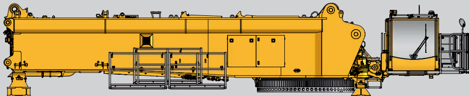
Transporteinheit Drehbühne Transport unit superstructure
